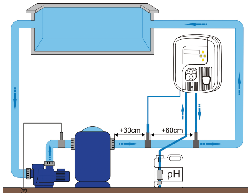
Installationschema pH clever:
