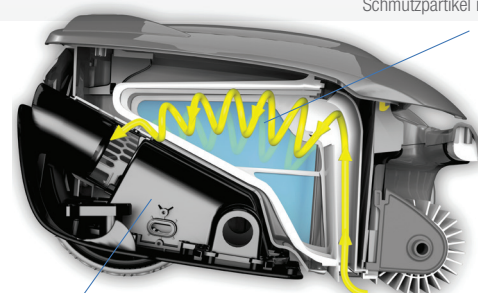
Geneigter Motor
