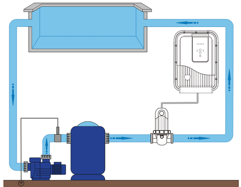
Installationsschema GenSalt OE:
